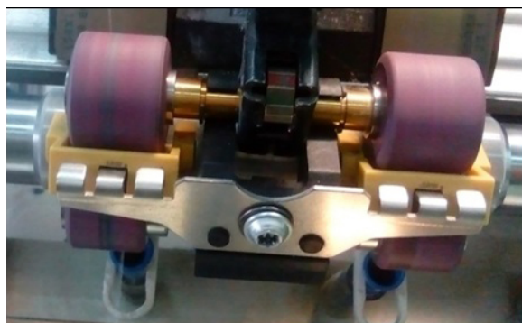
Fig. 1. Rotorcraft compact spinning roller (RoCoS).
